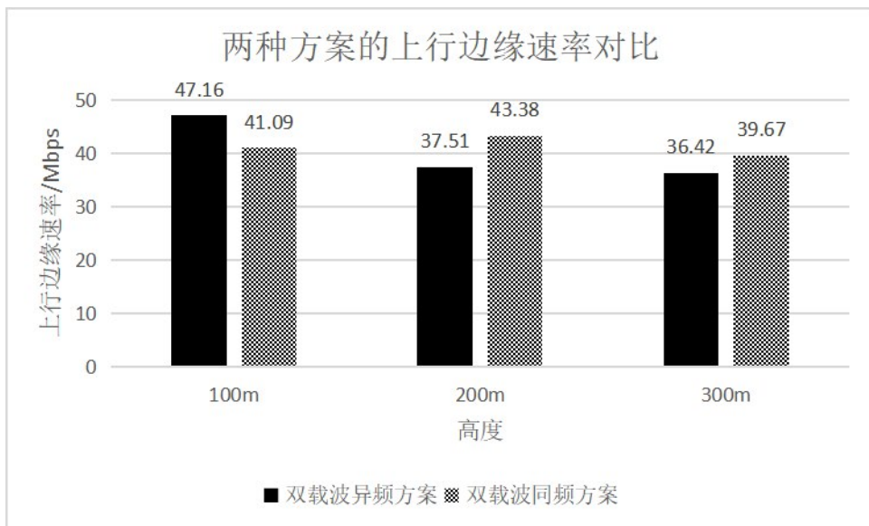
图 12 两种方案的上行边缘速率对比
