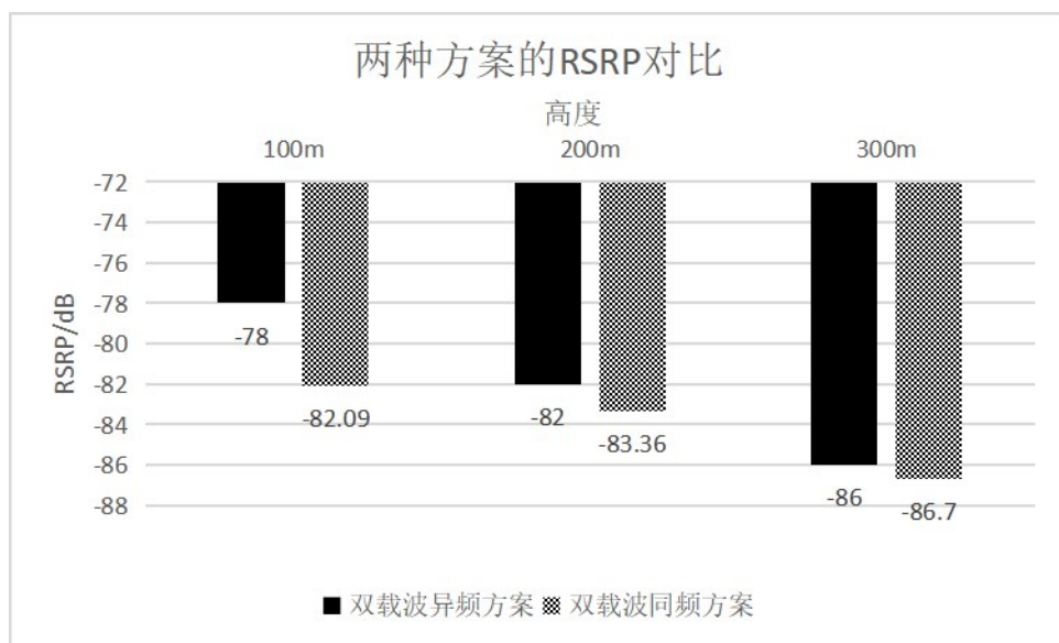
图10 两种方案测试结果RSRP对比
