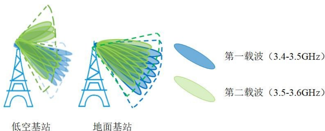
图4 双载波同频方案
