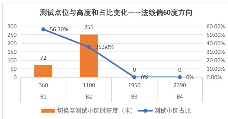
图 14 垂直起降法线偏 60 度方向测试结果
