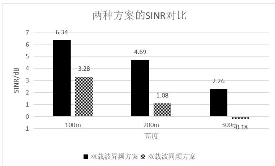
图 11 两种方案测试结果SINR 对比
