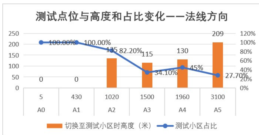
图 13 垂直起降法线方向测试结果
