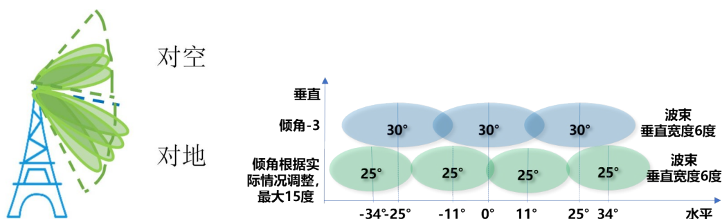
图2 3.5GHz 4+3 波束分层方案
